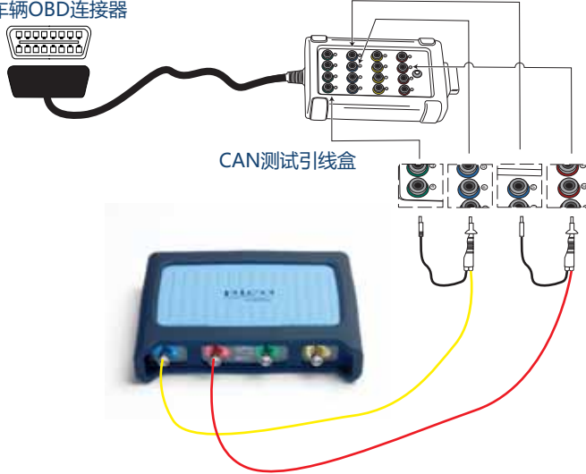
车辆OBD连接器
